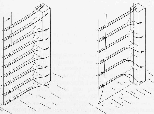
Bild 12. Übergeschwindigkeiten am Fusse eines Hochhauses
