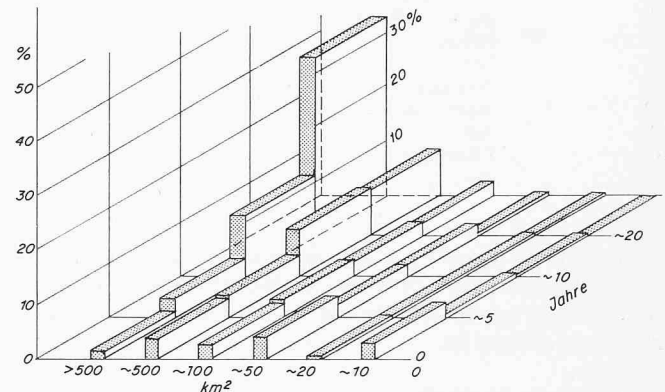
Bild 1. Aufteilung von 527 Abflussmess-Stationen der Schweiz nach Grösse des Einzugsgebietes und Beobachtungsdauer
