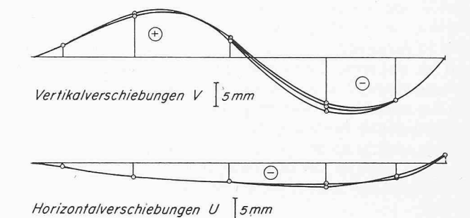
Bild 14. Gemessene Horizontal- und Vertikaldeformationen u und v für drei parallel liegende Messquerschnitte im Feld A (Lastfall 1)
