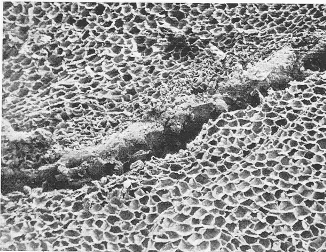
Bild 1. Kork (Backkork) mit versintertem Grenzgebiet zwischen zwei Schrotpartikeln; feinzellig
