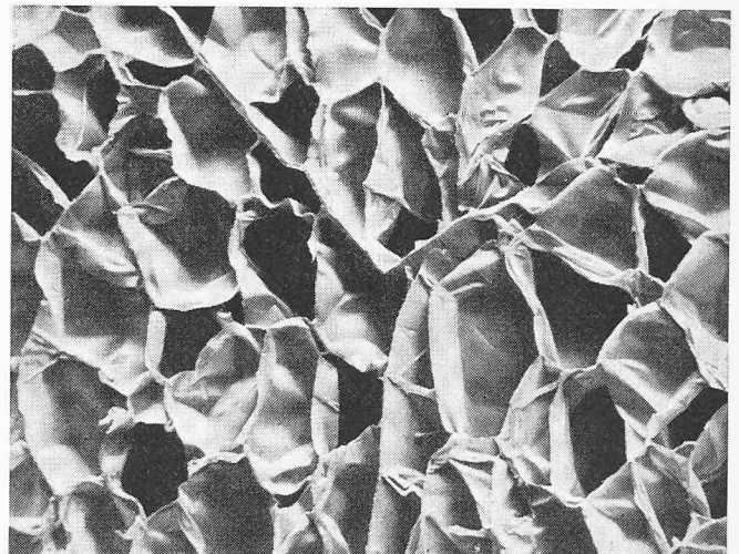
Bild 2. Polystyrol-Hartschaum (blockgeschäumt) im Grenzgebiet von drei verschmolzenen Partikeln; mittelgrosse Zellen
