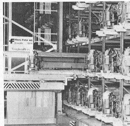
Bild 9. Webmaschine rollt automatisch vom Regalförderzeug in ein Lagerfach
