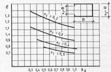
Bild 3. Einfluss der Raumgeometrie x_2 und der Ventilationsöffnungen x_1 auf die Auswirkung der Brandlast \epsilon
