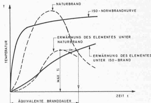
Bild 2. Ermittlung der äquivalenten Branddauer
