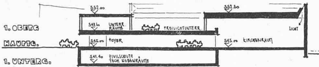
Schnitt durch Pfarrwohnungen 1:800
