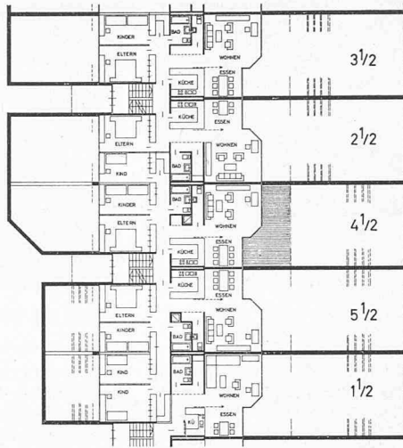
GRUNDRISEBENE B
