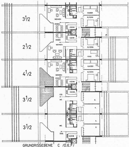
Grundriss 1:600
