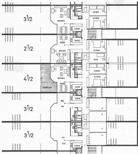
GRUNDRISEBENE B
