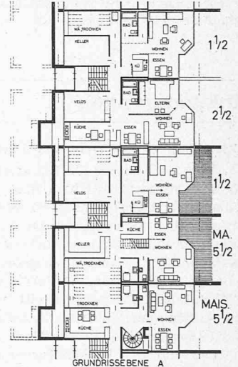
GRUNDRISEBENE A
