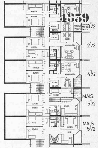
GRUNDRISEBENE B
