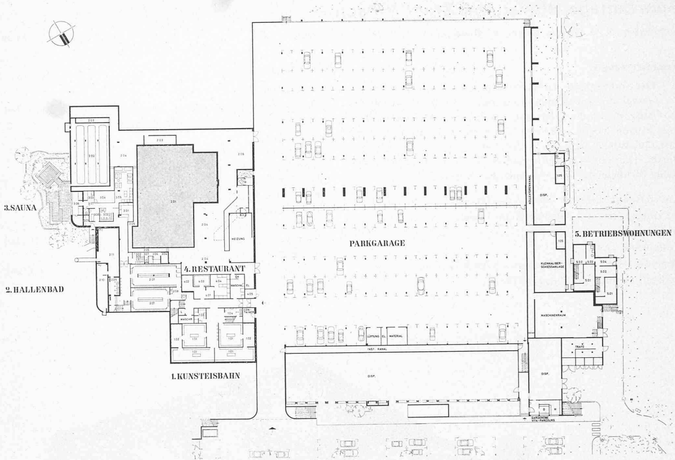
Grundriss Untergeschoss 1:900
