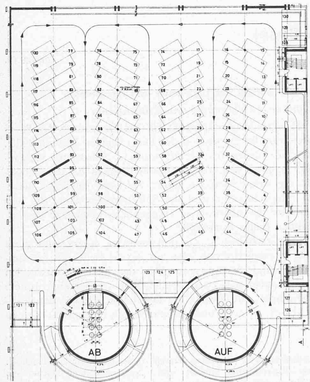
Grundriss Obergeschosse 1:800
