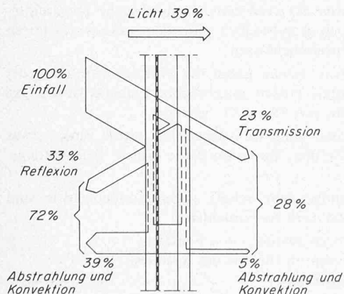
Energiebilanz von Infrastop-Auresin 39/28. 39% der Helligkeit (Licht) dringen in den Raum, aber nur 28% der Gesamtenergiemenge beeinflussen die klimatischen Bedingungen im Raum
