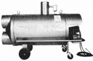
HATRA-Heissluft-Oelöfen für Grossraumheizung
