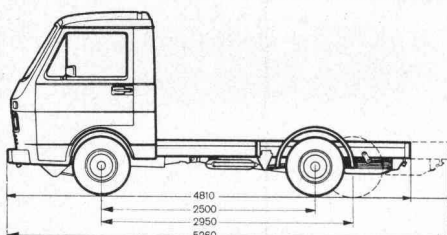
Chassiswagen.
