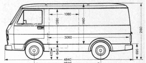
Kastenwagen.
