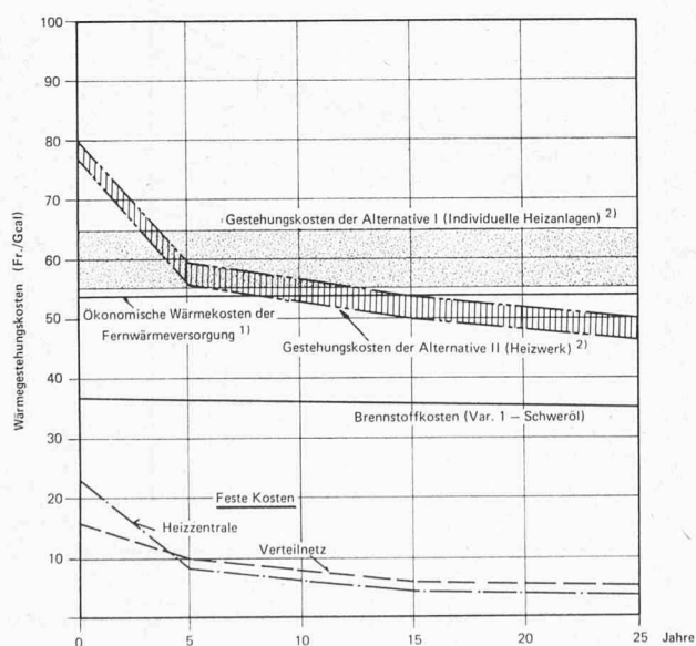
Bild 7. Gesteungskosten der Wärmeversorgung (Fallstudie)
