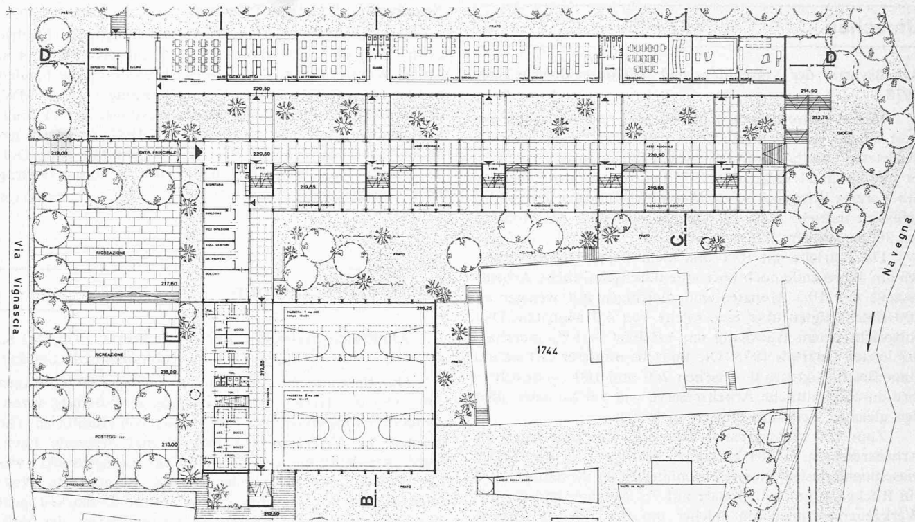
Grundriss Erdgeschoss 1:900
