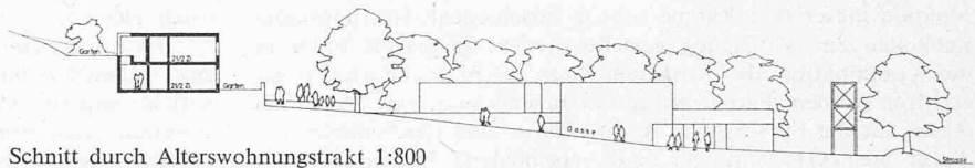
Schnitt durch Alterswohnungstrakt 1:800
