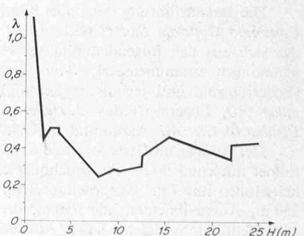
Bild 10. Verlauf des Seitendruckkoeffizienten an den Ulmen bei zunehmender Schütтарhöhe H (Mittel der gemessenen Seitendrücke)
