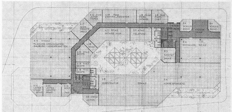
Grundriss 2. Obergeschoss 1:800
