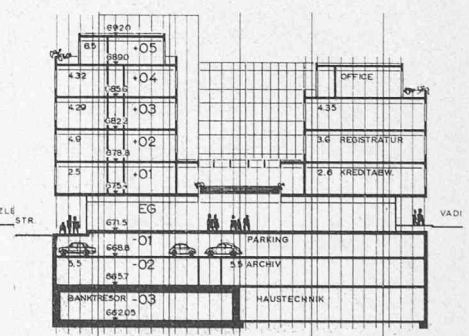
Querschnitt 1:800
