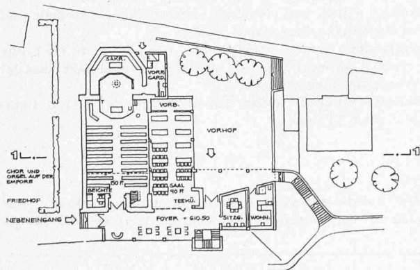
Erdgeschoss 1:800
