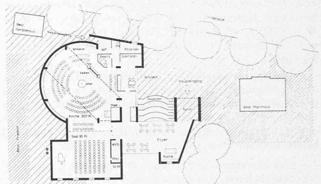
Erdgeschoss 1:800
