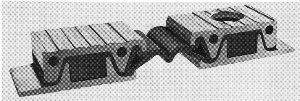
ELASTFUGE — eine vorgespannt verankerte, hochelastische Fahrfuge aus Aluminium-Neopren Verbundelementen.
