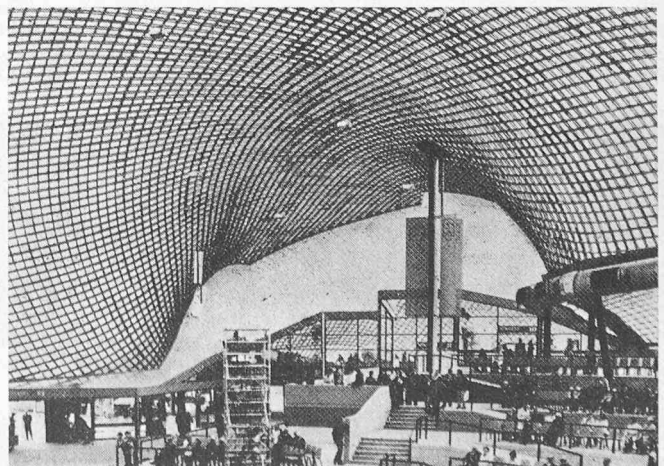
Bild 5. Innenansicht der Multihalle Mannheim (1975) [7]. Schalenförmiges Holzgitterdach aus total 72 km Holzlaten (5 × 5 cm). Der Gitterrost mit 50 cm Maschenweite wurde am Boden ausgelegt, dann bis zur gewünschten Höhe hochgehoben. Beim Hebevorgang verschoben und verformten sich die Latten, die in diesem Zeitpunkt nur lose an den Kreuzungsstellen zusammengehalten wurden. Dann aber wurden die 8-mm-Schraubbolzen angezogen, und die Ränder der Gitterschale wurden an die Brettstapelverleimten Randträger angeschlossen. Überdachte Fläche 7400 m 2 , Kuppelhöhe max. 20 m
