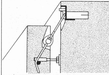
Edelstahl-Anker, -Schienen und Zubehör Verbund-, Zug- und Windanker Betonfertigteil-Transportringanker
