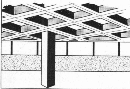
Kassetten- und Rippendecken-Schalkörper Verdrängungskörper und Schalelemente Bauwerks-Einstiegsöffnungen
