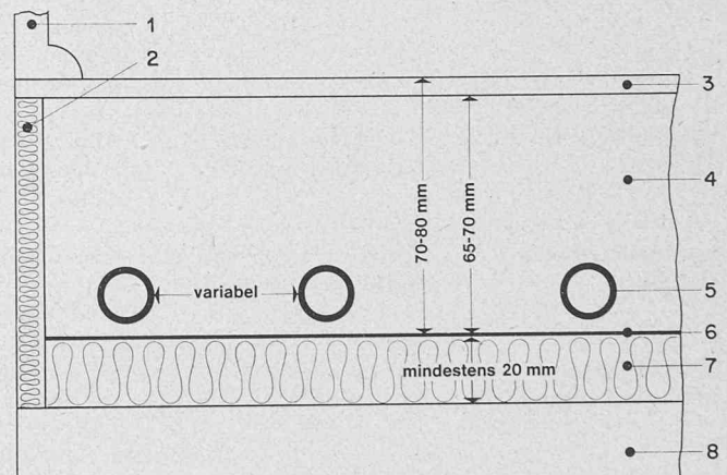
Multibetonssystem im Detail. 1 Fussleiste, 2 Randstreifen, 3 Bodenbelag, 4 Unterlagsboden, 5 Multibeton-Rohr, 6 Baufolie, 7 Wärmeisolierung, 8 Betondecke
