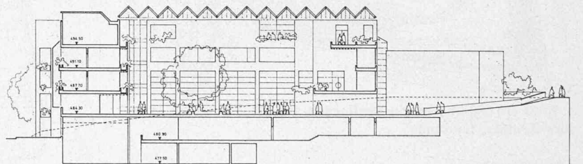
Schnitt Studios-Zugangsrampe 1:750
