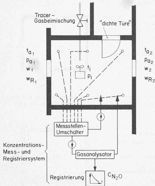
Bild 3. Messeinrichtung zur Bestimmung des Luftwechsels in einem unbewohnten Zimmer mit gegenüberliegenden angeordneten Aussenfenstern und gut dichter Türe
