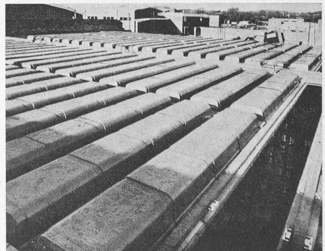
Bild 9. Wiedergewinnbare Rippendeckenschalung
