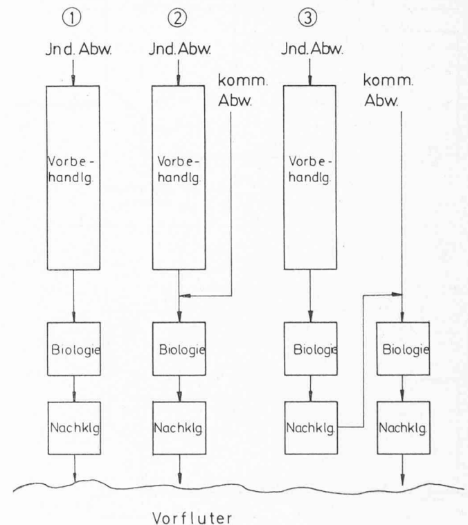
Bild 1. Kombinationsmöglichkeiten von Industrie- und Kommunabwasser
