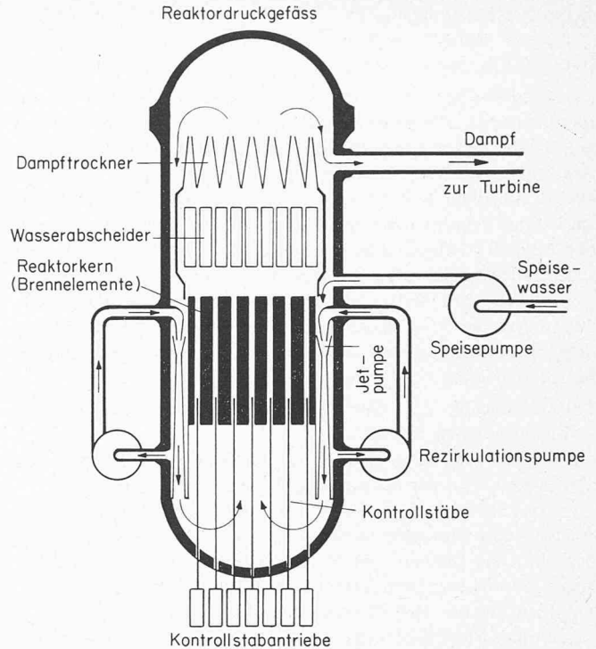
Bild 2. Siedewasser-Kreislaufschema
