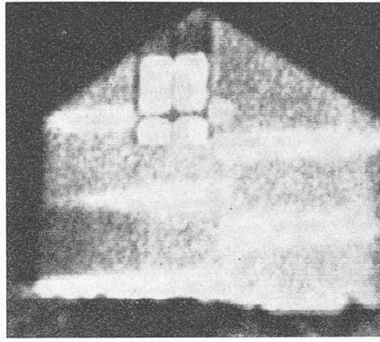
Bild 9 (links). Isolationstechnisch einwandfreie Fassade. – Bild 10 (Mitte). Massive Wärmeverluste durch mangelhafte Isolation von Betondecken. – Bild 11 (rechts). Sichtbarmachung von Riegelwerk, welches dem blossen Auge durch eine Putzschicht verdeckt bleibt
