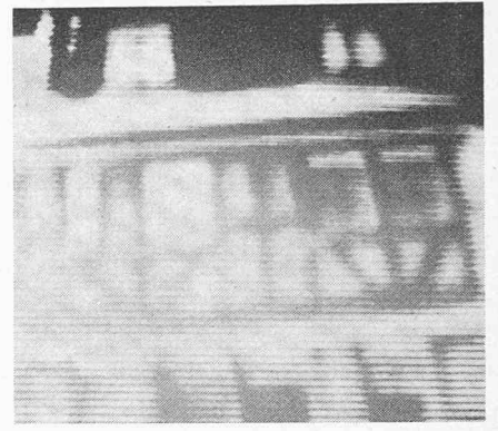
Bild 9 (links). Isolationstechnisch einwandfreie Fassade. – Bild 10 (Mitte). Massive Wärmeverluste durch mangelhafte Isolation von Betondecken. – Bild 11 (rechts). Sichtbarmachung von Riegelwerk, welches dem blossen Auge durch eine Putzschicht verdeckt bleibt
