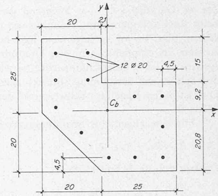
Bild 8. Eckpfeiler
