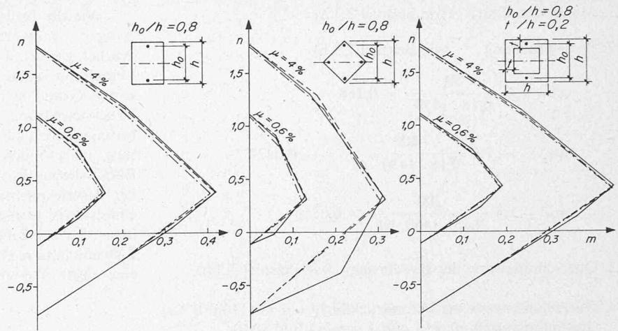
Bild 12. Interaktionsdiagramm der Bruchschnittkräfte. Vergleich verschiedener Berechnungsannahmen. Ausgezogene Linien: Dehnungsverteilung nach Bild 10a, Betonspannungen nach Gl. (8). Strichpunktete Linien: Dehnungsverteilung nach Bild 10b, Betonspannungen nach Gl. (8). Gestrichelte Linien: Dehnungsverteilung nach Bild 10b, rechteckiger Spannungsblock nach Bild 11
