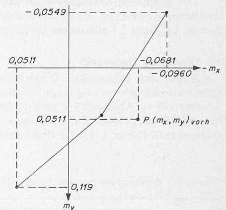
Bild 9. Interaktionsdiagramm der zulässigen Schnittkräfte für den allgemeinen Querschnitt
