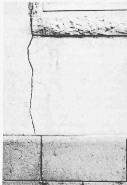
Bild 5. Thermische Risse
