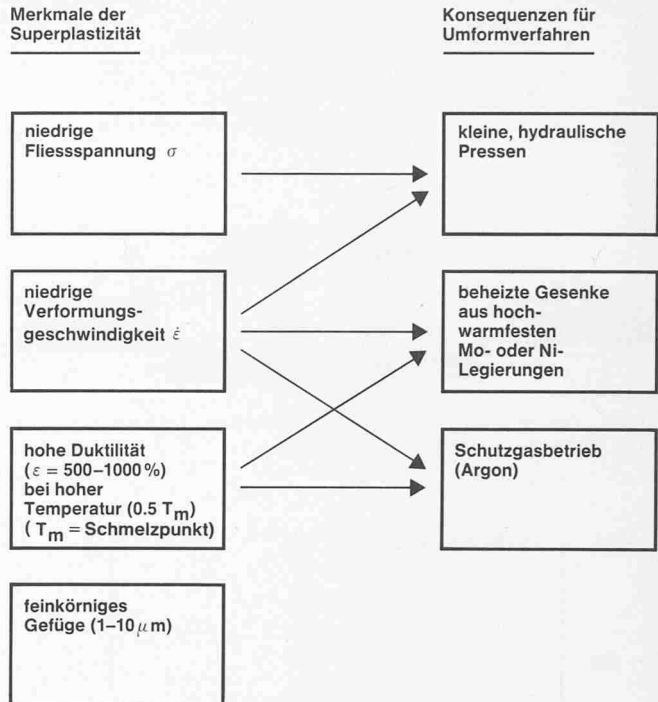
Bild 3. Merkmale der Superplastizität und Konsequenzen für Umformverfahren
