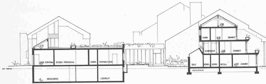
SCHNITT B-B
