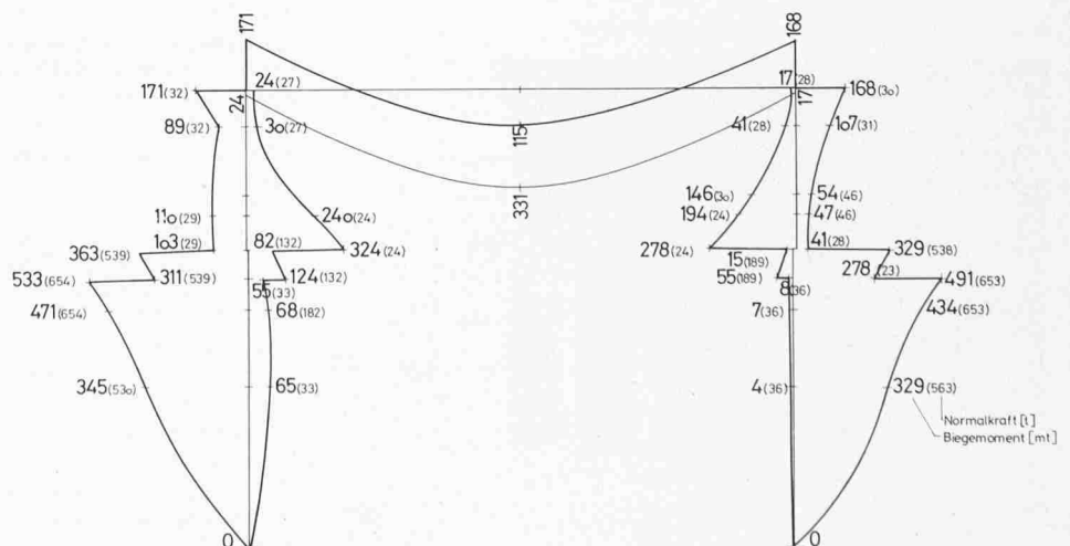
Bild 8. Grenzwertlinien Hauptrahmen
