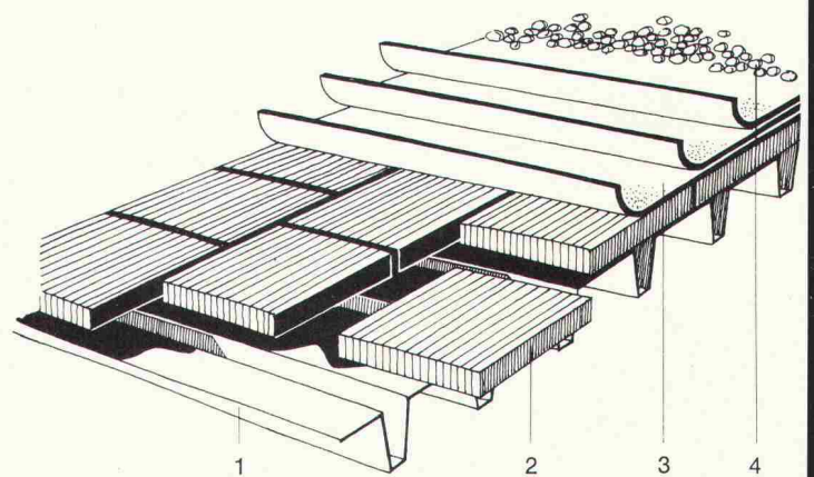
METALLPROFILDACH
