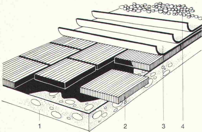
BETONFLACHDACH
