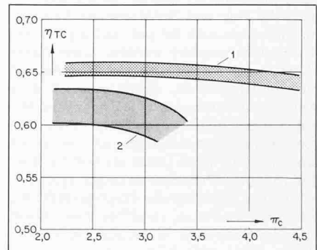
Bild 2. Turboladerwirkungsgrad, Vergleich VTR 454/VTR 501. \eta_{TC} : Gesamtwirkungsgrad des Turboladers (Bereiche für verschiedene Turboladerspezifikationen), \pi_C : Verdichterdrukverhältnis (1 VTR 454, 2 VTR 501, in Produktion seit 1970, Wirkungsgraderhöhung seit 1975)
