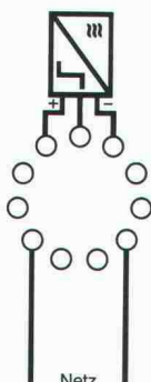
Elektronische Zeitrelais multiCOMAT RS 121
