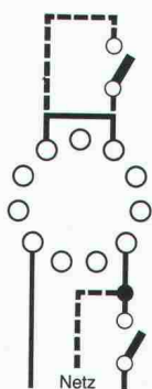
Elektronische Zeitrelais multiCOMAT RS 121
