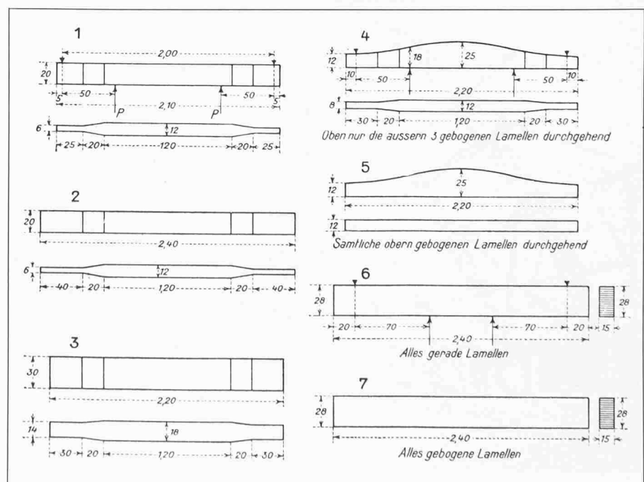
Bild 11. Durch F. Hübner an der EMPA Zürich untersuchte Typen verleimte Biegebalken, 1919 [7]
