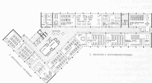
Grundriss 2. Obergeschoss 1:1000
