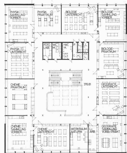
Grundriss 2. Obergeschoss 1:650
