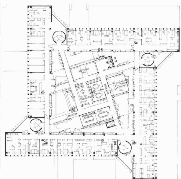
Grundriss 1.-5. Obergeschoss, Variante 2, 1:750 Rechts: Grundriss Untergeschoss 1:750
