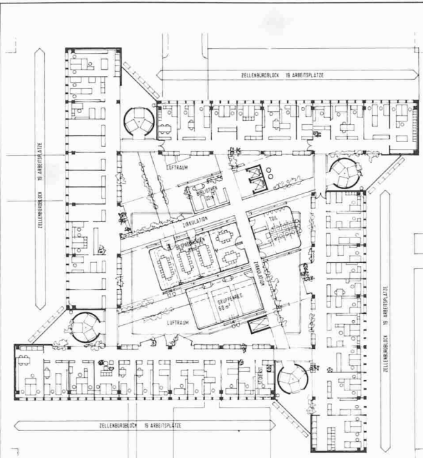
Grundriss 1.-5. Obergeschoss, Variante 1, 1:750 Rechts: Grundriss Erdgeschoss 1:750
