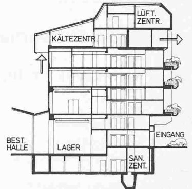
Schnitt Eingangspartie 1:750
