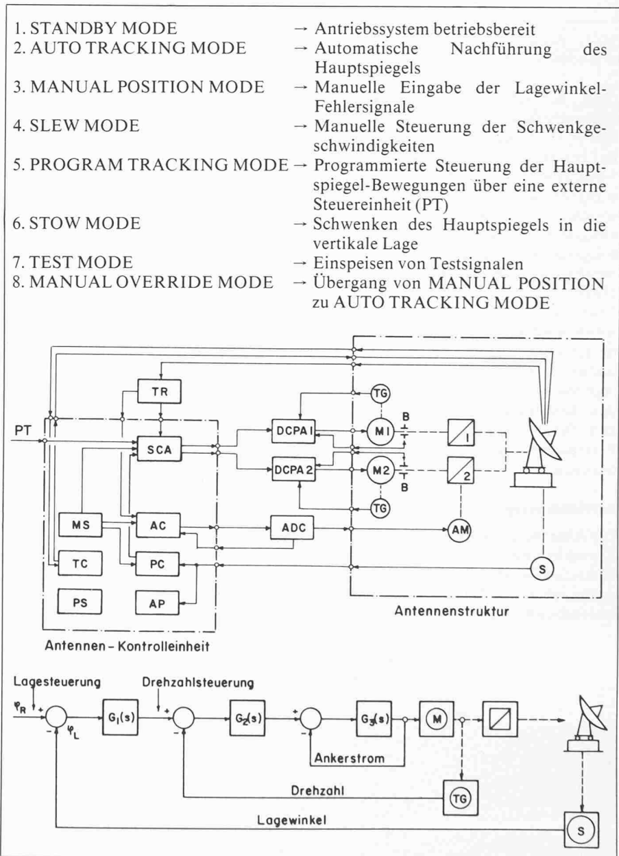
Bild 8. Vereinfachte Blockschemata der Steuerungs- und Servosysteme (nur eine Achse dargestellt)
