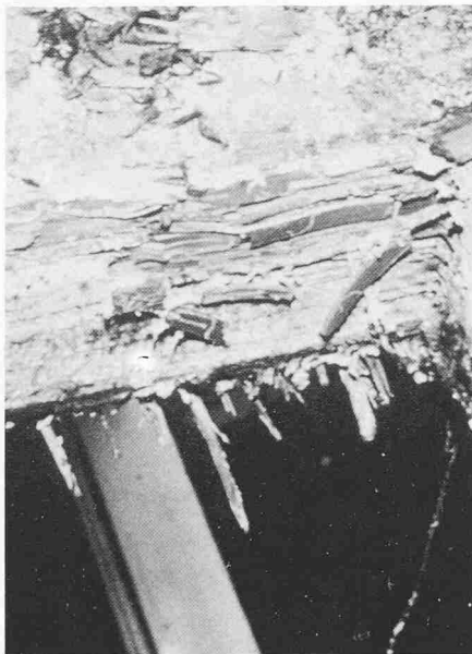
Bild 3. Durch den Balkenblättling ( Gloeophyllum trabeum Murrill) zerstörter Balken
