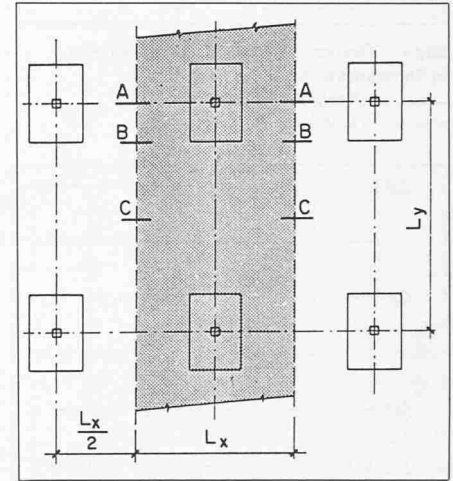
Bild 2. Verlauf der Biegemomente. Grundriss
