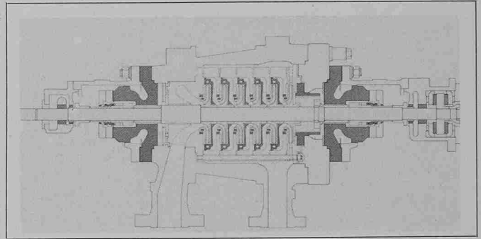
Schnitt einer mehrstufigen Sulzer Mantelgehäusepumpe Typ GSG
