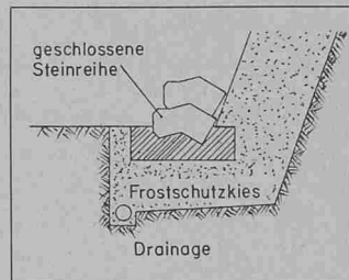
Ausbildung des Fusspunktes bei waserdurchlässigem Untergrund
