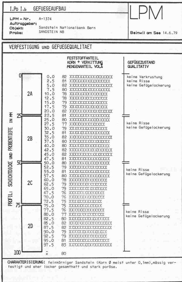
Bild 9. Profilanalyse Mengenteilung einer Gefügekomponente über ein bestimmtes Profil im Baustoff Beispiele: - Bindemittelanteil und Verteilung - Zuschlagverteilung - Homogenität - Porenanteil und Verteilung - Profilaufzeichnung eines Gefügeanteils, Auflockerung, Auslaugung, Zerfall oder Entmischung usw.
