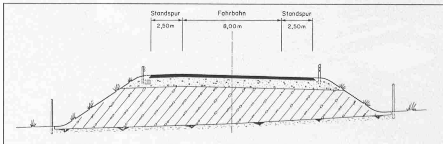
Normalprofil Autostrasse
