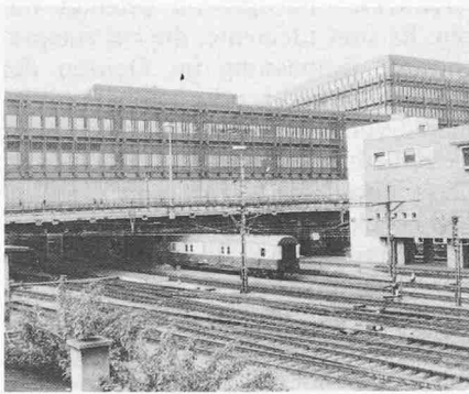
Überdeckung von Perrons und Geleisen durch mehrgeschossigen Betriebsbau. Postzentrum Basel über Bahnhof SBB
