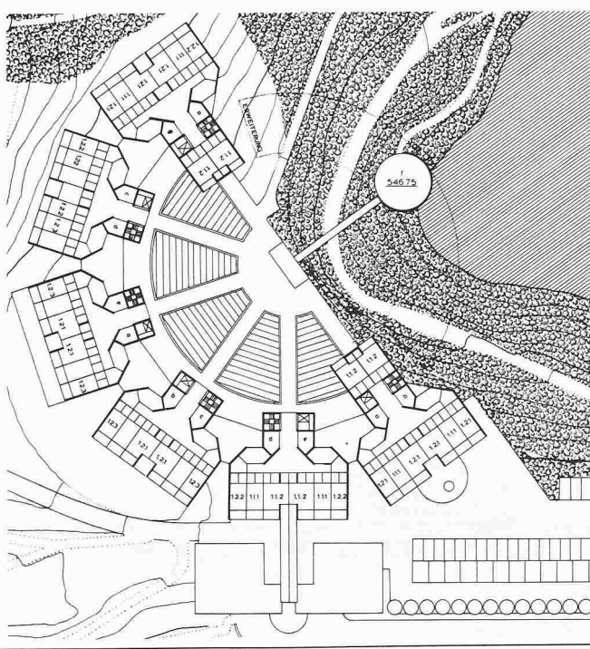
Grundriss Obergeschoss 1:1500
