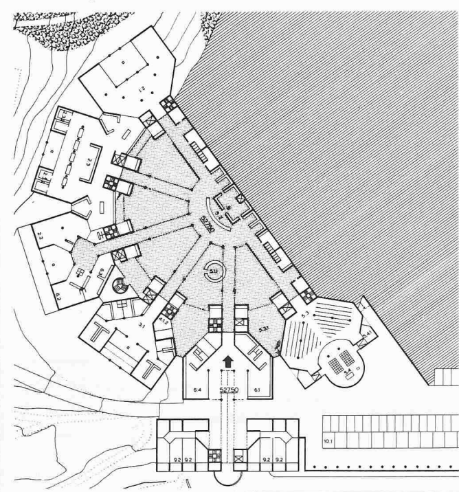
Grundriss Erdgeschoss 1:1500
