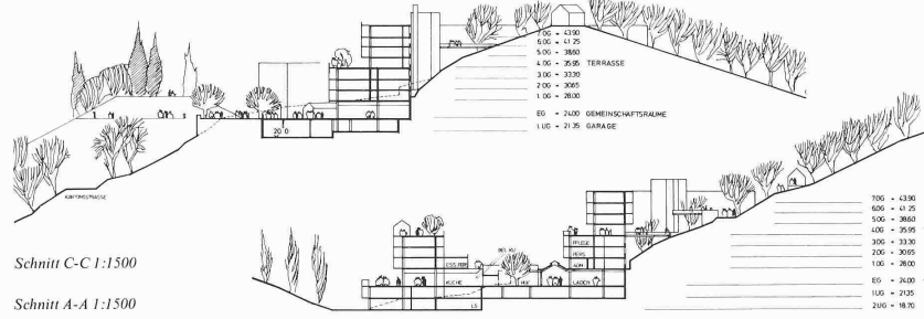
Schnitt A-A 1:1500
